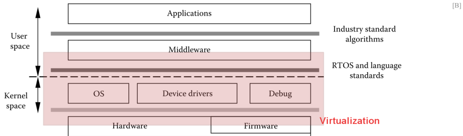
Abb. 12. Typische Datenverarbeitungsebenen in Eingebetteten Systemen und Virtualisierung
