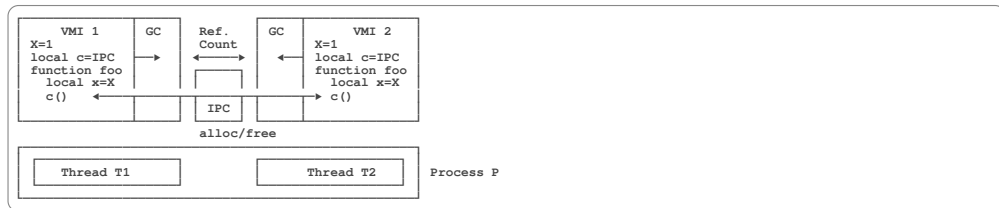
Abb. 25. Zwei Lua LVM Instanzen mit gemeinsamen eng gekoppelten Interprozeßkommunikationsobjekten und implizite GC Kopplung über Referenzzählung
