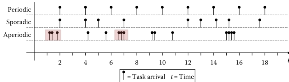
Abb. 23. Periodische, sporadische, und aperiodische Tasks
