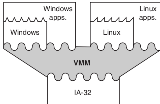
Abb. 4. Beispiel: Zwei Betriebssysteme werden auf virtualisierter Hardware (parallel) ausgeführt
