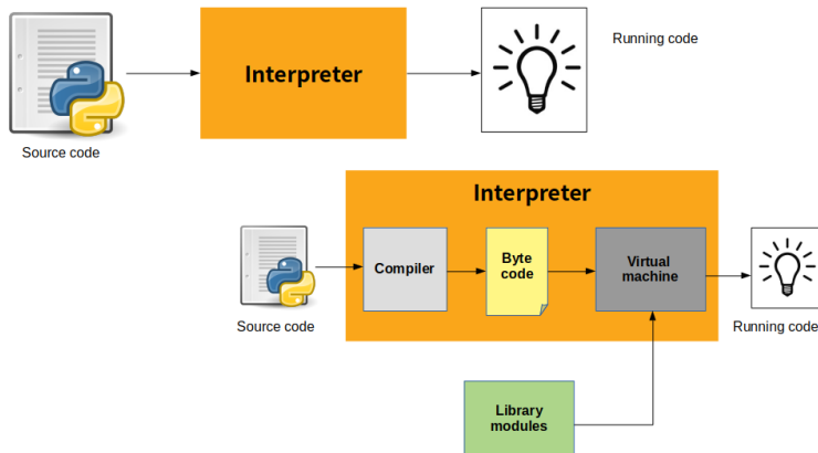
Abb. 7. Vergleich Interpreter mit Bytecode Compiler-Interpreter System
