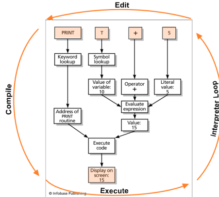
Abb. 6. Edit - Compile - Execute Zyklus bei einem Interpreter
