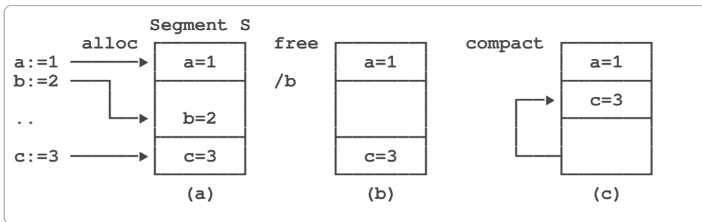
Bsp. 3. (a) Speicherbelegung, (b) Freigabe, und (c) Kompaktierung
