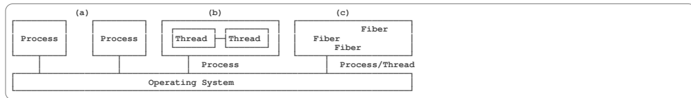
Abb. 18. (a) Zwei isolierte Prozess (b) Zwei gekoppelte Threads in einem Prozess (c) Koroutine (Fibers), nicht isoliert mit einem Kontrollpfad
