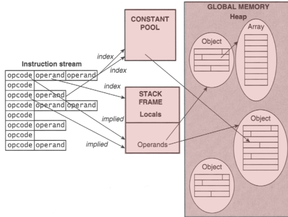
Abb. 15. Speicherhierarchie von Programmen und Zusammenhang mit Maschinenanweisungen
