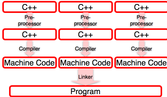
Abb. 5. Klassischer Softwareentwurf mit Compiler und Linker (C)
