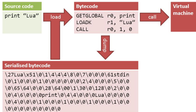
Abb. 9. Bytecode VM
